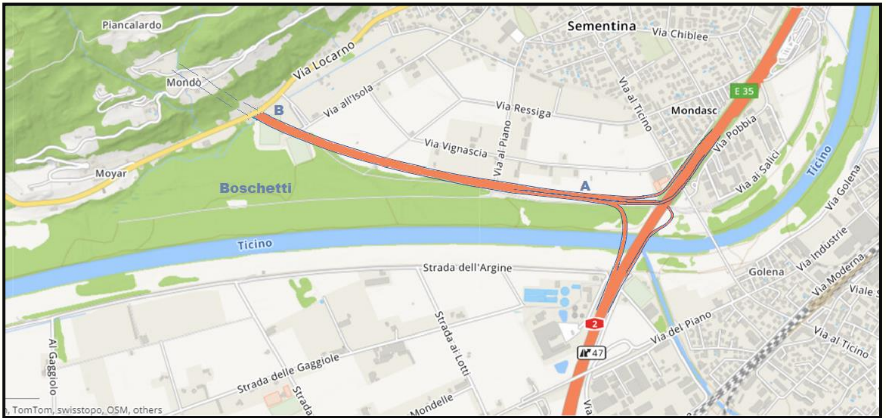
Allacciamento autostradale A2 - A13 Variante sponda destra La diramazione di Sementina (Da A a B il tracciato è in galleria artificiale coperta)
