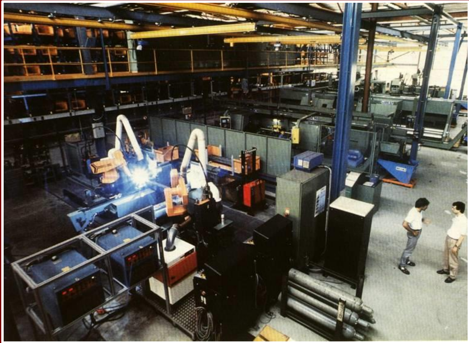
Robots soudeurs en action
